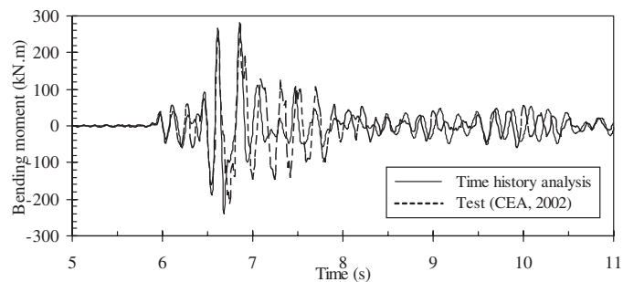
(d) Bending moment at level 1
